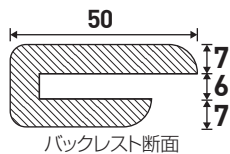
バックレスト断面
